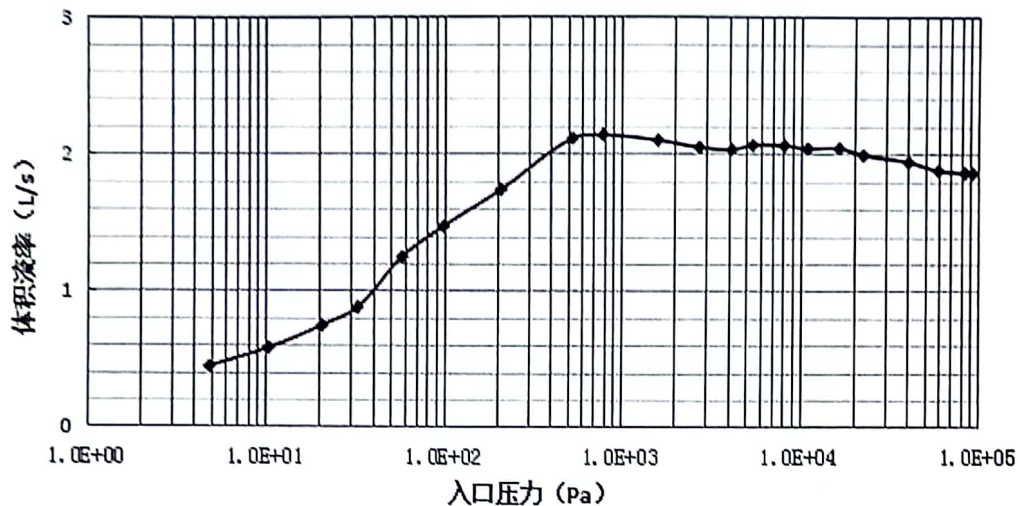
入口压力、体积流率-曲线
