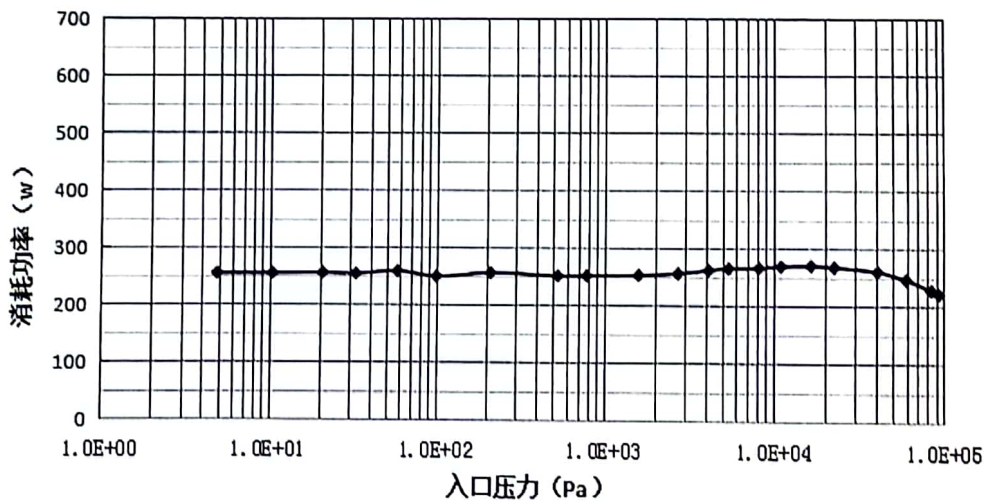
入口压力、消耗功率-曲线
